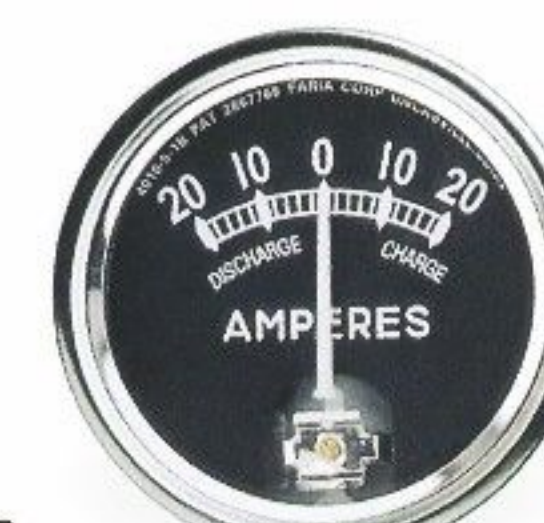
φ 52 ±20A AMMETER
